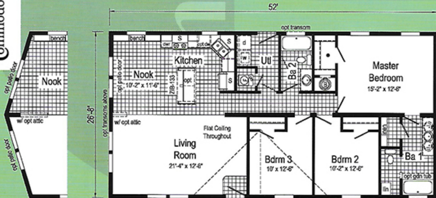
Optional Prow End
