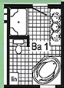
Optional Glamour Bath (omits linen closet)
